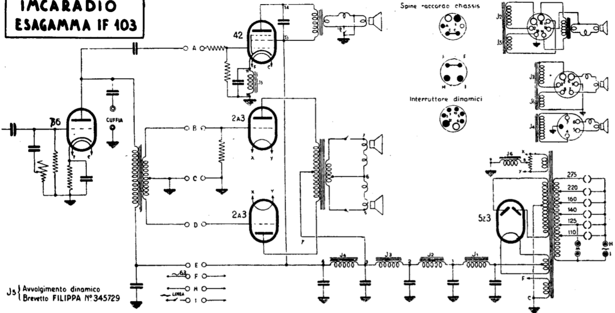
63. — IMCARADIO. — Esagamma I F 103. — A canali indipendenti (Brev. Fonorilievo), — Produzione 1938-39.
